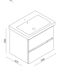
Vega Banyo Dolabı 60 Vega Bathroom Cabinet 60 Vega Badezimmerschrank 60
