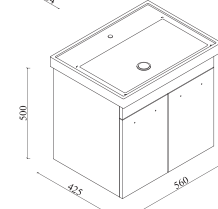
Nil Banyo Dolabı 60 Nil Bathroom Cabinet 60 Nil Badezimmerschrank 60
