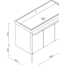
Karina Banyo Dolabı 100 Karina Bathroom Cabinet 100 Karina Badezimmerschrank 100
