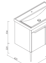
Karina Banyo Dolabı 80 Karina Bathroom Cabinet 80 Karina Badezimmerschrank 80
