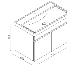
Arya Banyo Dolabı 80 Arya Bathroom Cabinet 80 Arya Badezimmer Schrank 80
