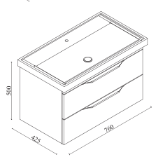
Lotus Banyo Dolabı 80 Lotus Bathroom Cabinet 80 Lotus Badezimmerschrank 80
