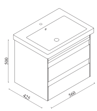
Lara Banyo Dolabı 60 Lara Bathroom Cabinet 60 Lara Badezimmerschrank 60
