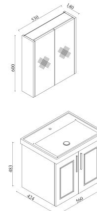
Arin Banyo Dolabı 60 Arin Bathroom Cabinet 60 Arin Badezimmerschrank 60
