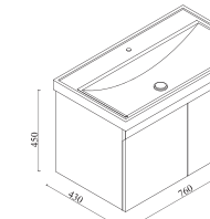
Alfa Banyo Dolabı 80 Alfa Bathroom Cabinet 80 Alfa Badezimmerschrank 80
