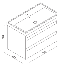
Lara Banyo Dolabı 80 Lara Bathroom Cabinet 80 Lara Badezimmerschrank 80
