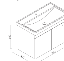
Nil Banyo Dolabı 80 Nil Bathroom Cabinet 80 Nil Badezimmerschrank 80
