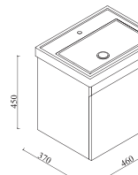
Alfa Banyo Dolabı 50 Alfa Bathroom Cabinet 50 Alfa Badezimmerschrank 50
