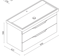
Lotus Banyo Dolabı 100 Lotus Bathroom Cabinet 100 Lotus Badezimmerschrank 100
