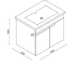
Gonca Banyo Dolabı 65 Gonca Bathroom Cabinet 65 Gonca Badezimmerschrank 65
